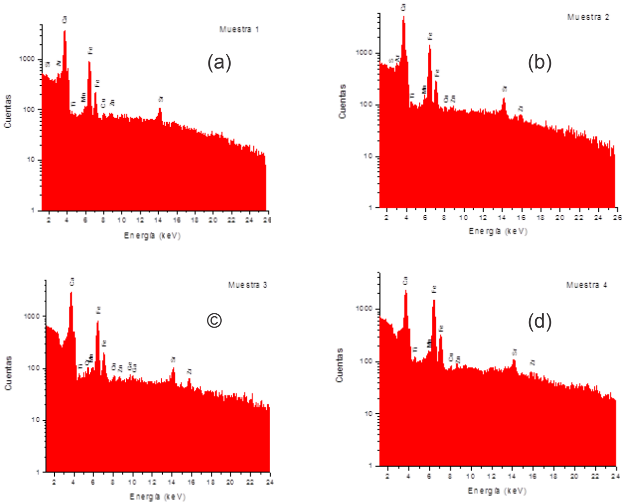
Figura 7. Espectros de fluorescencia de rayos X por energía dispersiva de las muestras (a) muestra 1, (b) muestra 2, (c) muestra 3 y (d) muestra 4; de sedimentos de la laguna El Paraíso.
