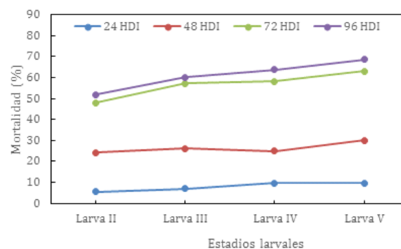
Figura 1. Mortalidad (%) de S. frugiperda según estadio larval y horas después de la inoculación (HDI).
