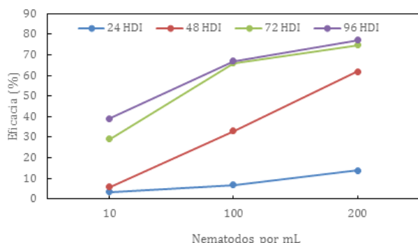
Figura 4. Eficacia de control (%) de S. frugiperda según concentraciones de H. bacteriophora y horas después de la inoculación (HDI).
