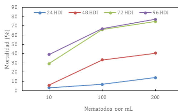
Figura 2. Mortalidad (%) de S. frugiperda según concentraciones de H. bacteriophora y horas después de la inoculación (HDI).
