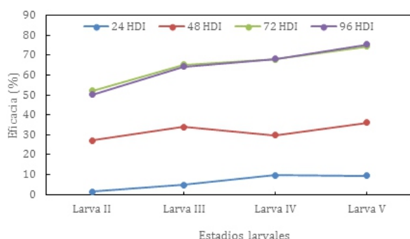
Figura 3. Eficacia de control (%) de S. frugiperda según estadio larval y horas después de la inoculación (HDI).
